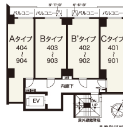
基準階平面図
